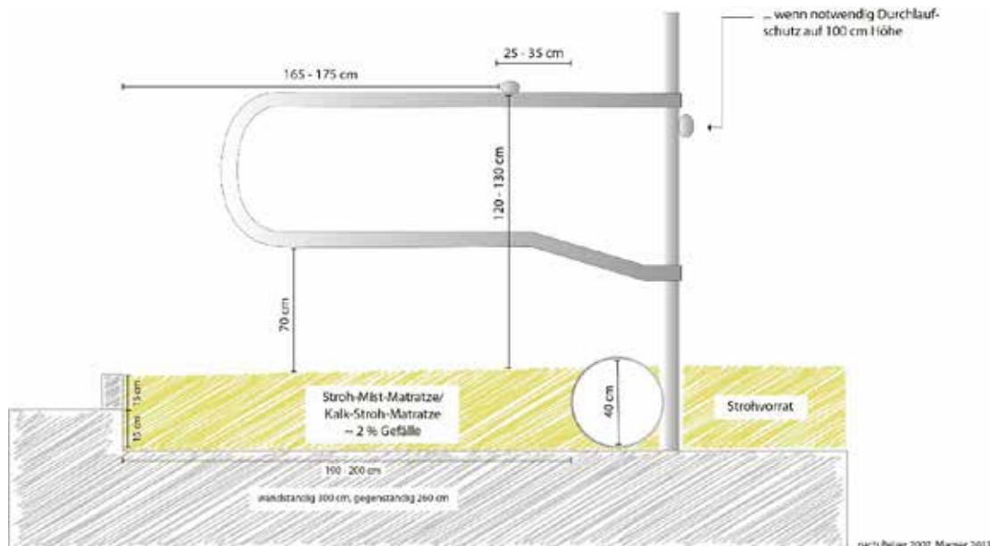
Die wichtigsten Abmessungen für eine gut eingestellte Liegebox.
